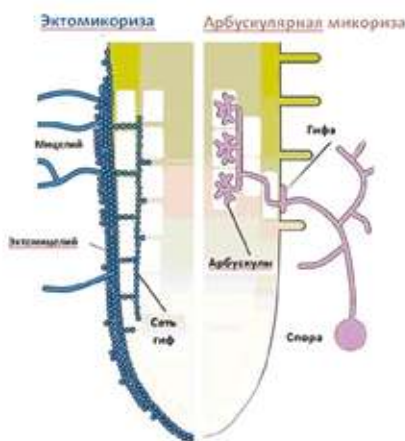
Рис. 1. Различия взаимодействия с корнем АМ и ЕСМ микоризы.
