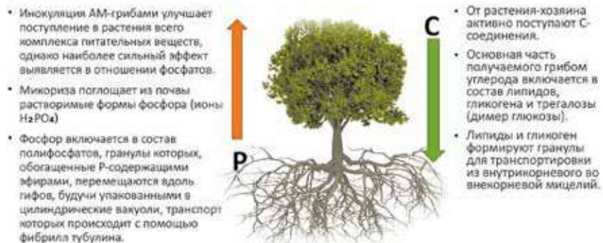
Рис.3 H_2PO_4
